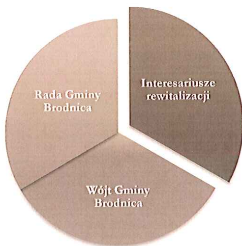
Schemat 3. Podmioty uczestniczące w realizacji programu rewitalizacji
