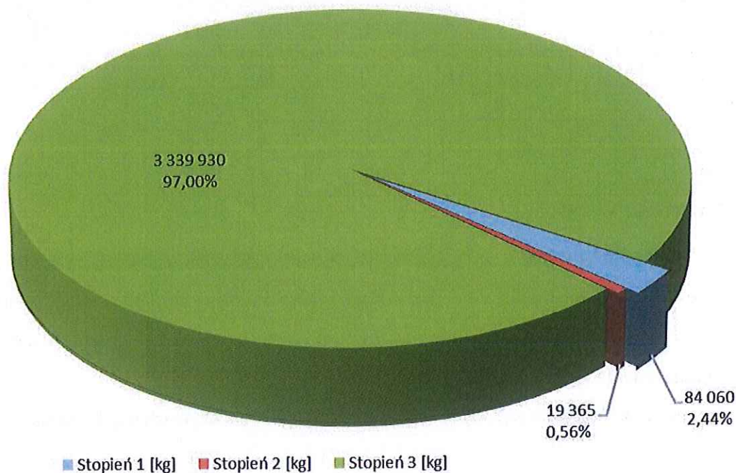
Rysunek 7. Ilość wyrobów zawierających azbest w podziale na stopnie pilności usunięcia w Gminie Brodnica.
